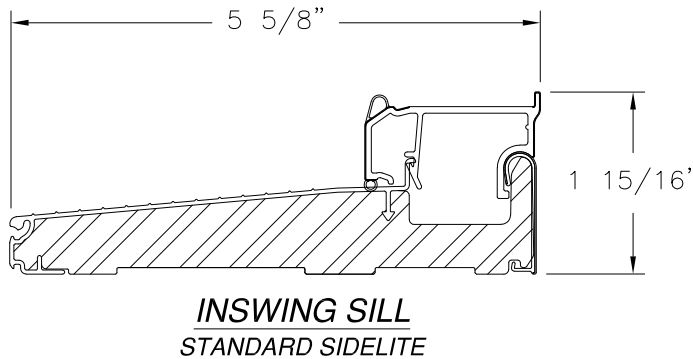
INSWING SILL DOOR
