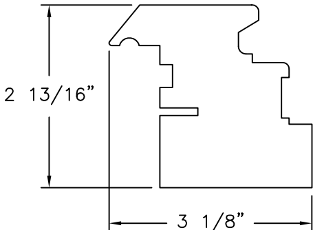
— SASH RIGHT JAMB (FRENCH OAK)
