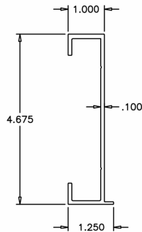
4 FRAME JAMB
