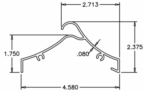
1 LOUVER BLADE
