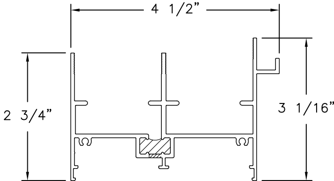
JAMB (BAM-1004) ALUMINUM 6063-T6
