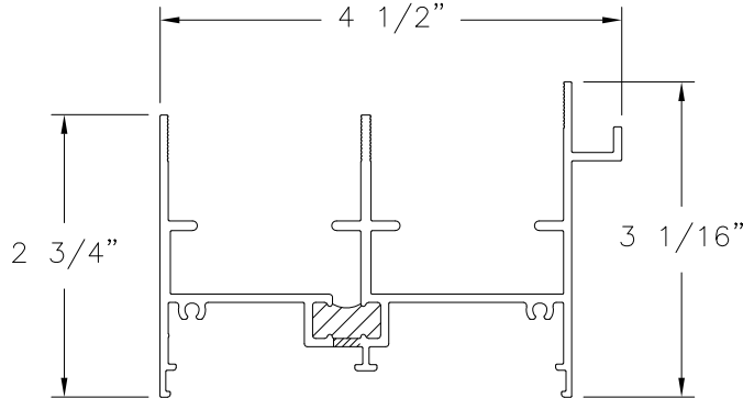
JAMB (BAM-1004) ALUMINUM 6063-T6
