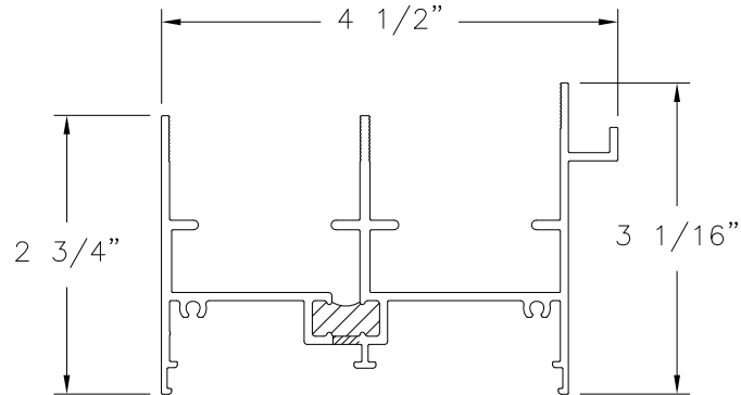
JAMB (BAM-1004) ALUMINUM 6063-T6
