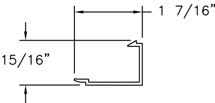
TRIM BASE (WLB-2005) ALUMINUM 6063-T5
