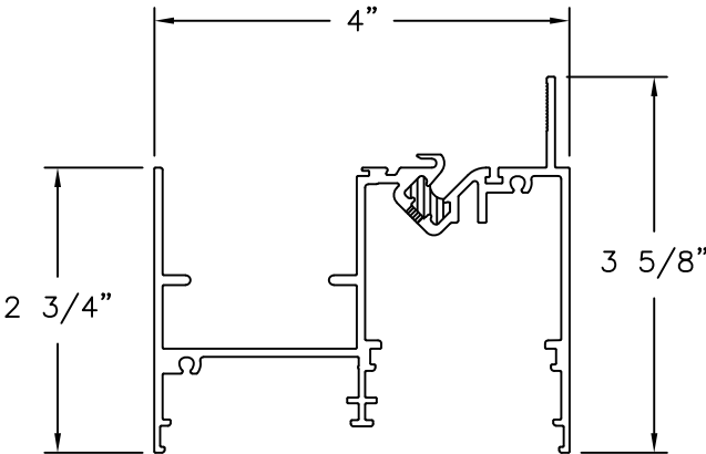
JAMB (BAM-1003) ALUMINUM 6063-T6
