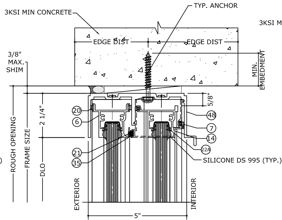
1.1A HEAD DETAIL (CONCRETE) N.T.S
