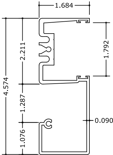
1 JAMB
