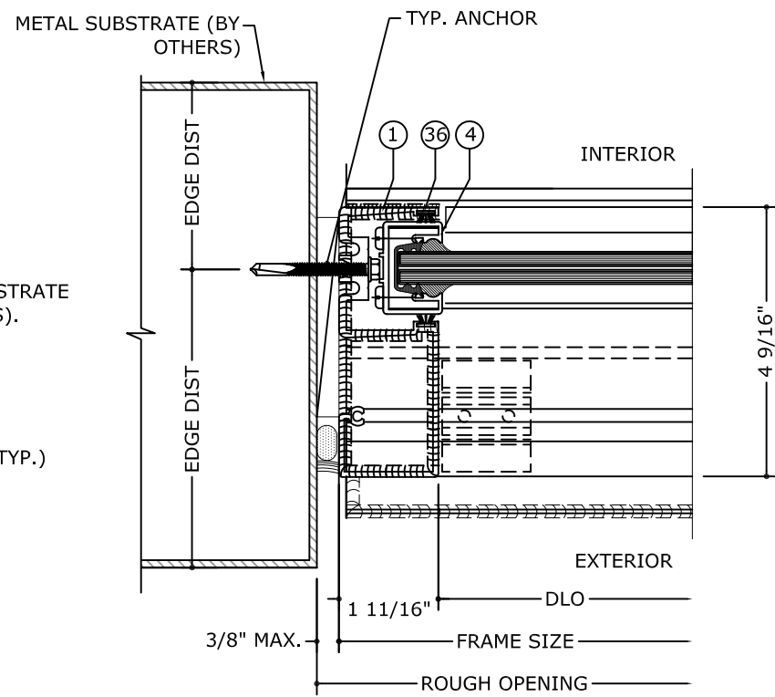
3.5 FIXED JAMB DETAIL (METAL) N.T.S.
