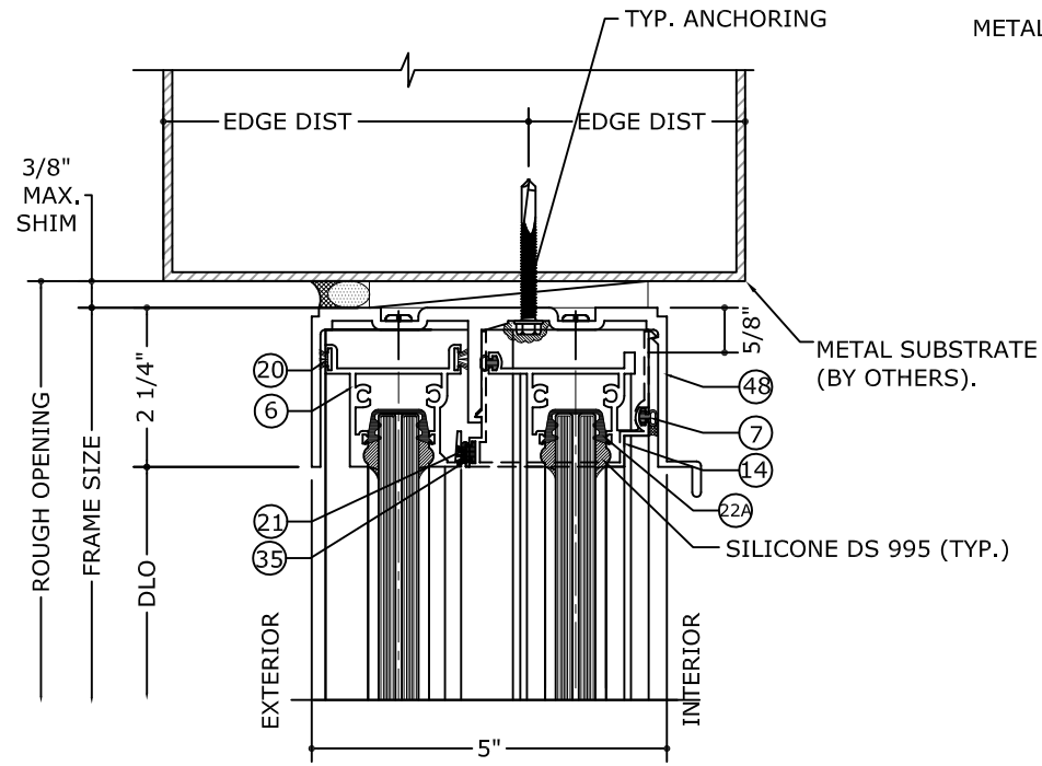
1.3A HEAD DETAIL (METAL) N.T.S.
