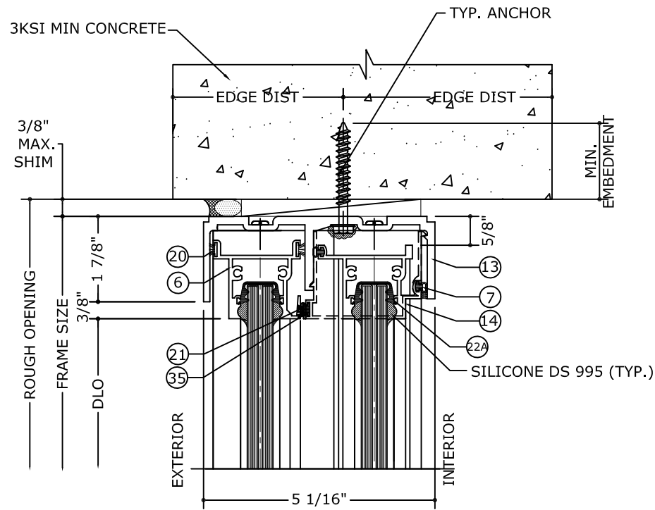
1.1 HEAD DETAIL (CONCRETE) N.T.S
