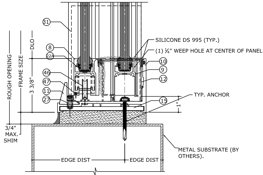
2.3 SILL DETAIL (METAL) N.T.S.
