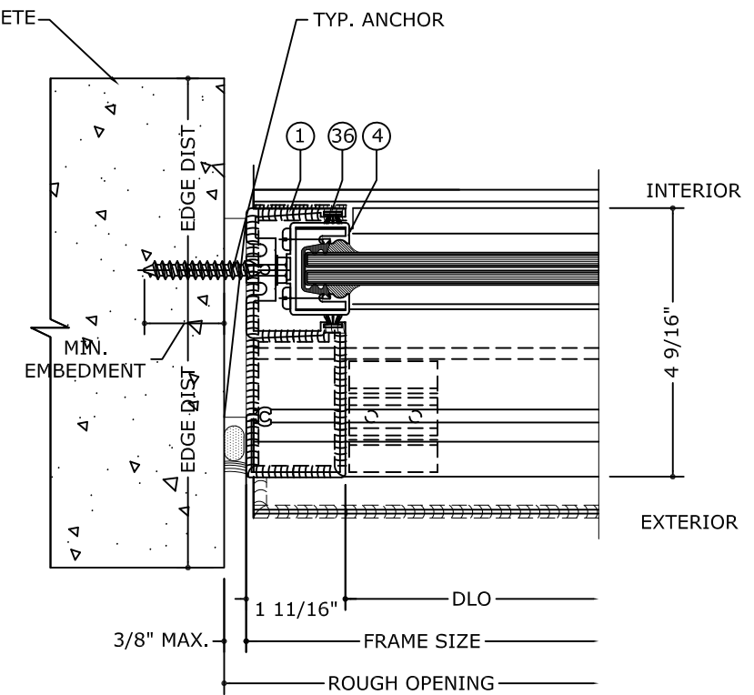
3.1 FIXED JAMB DETAIL (CONCRETE) N.T.S
