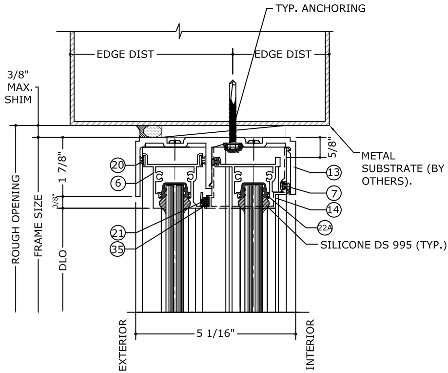
1.3 HEAD DETAIL (METAL) N.T.S.
