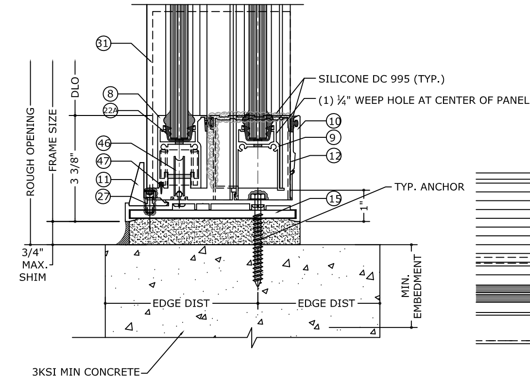
2.1 SILL DETAIL (CONCRETE) N.T.S
