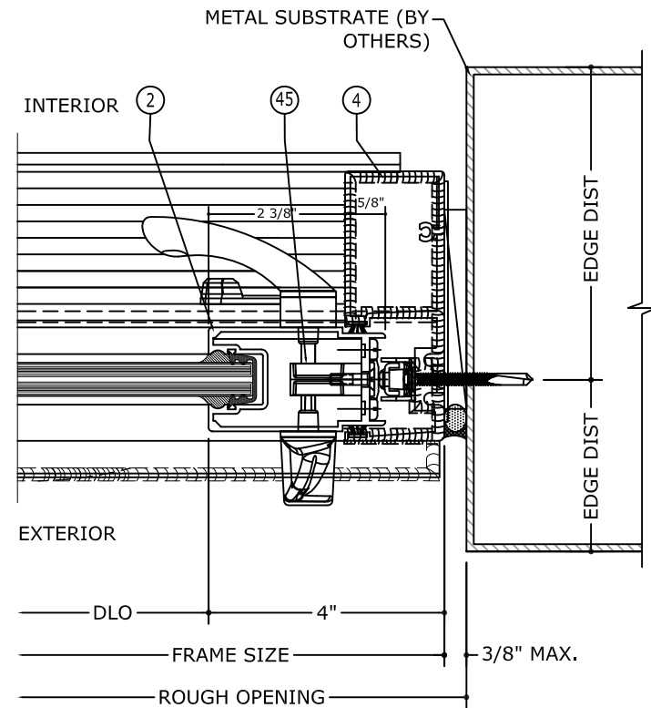
4.3 OPERABLE JAMB DETAIL (METAL) N.T.S.
