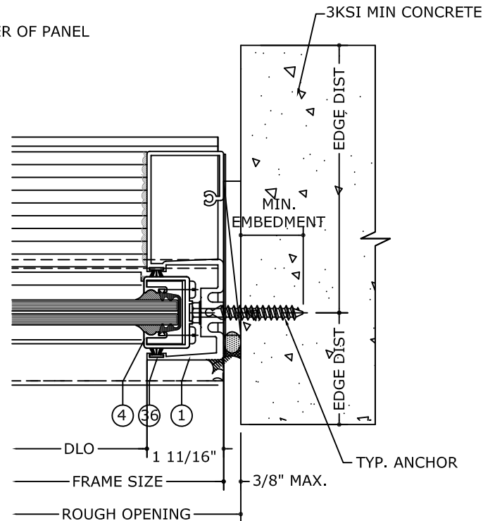
3.2 FIXED JAMB DETAIL (CONCRETE) N.T.S
