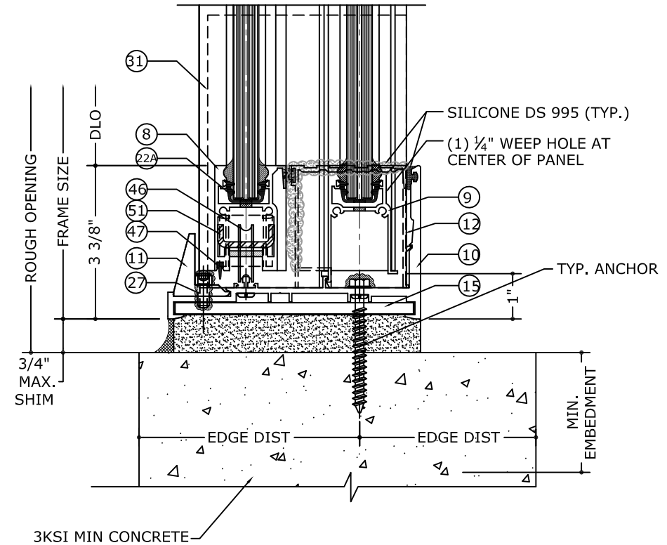
7 SILL DETAIL (CONCRETE) N.T.S
