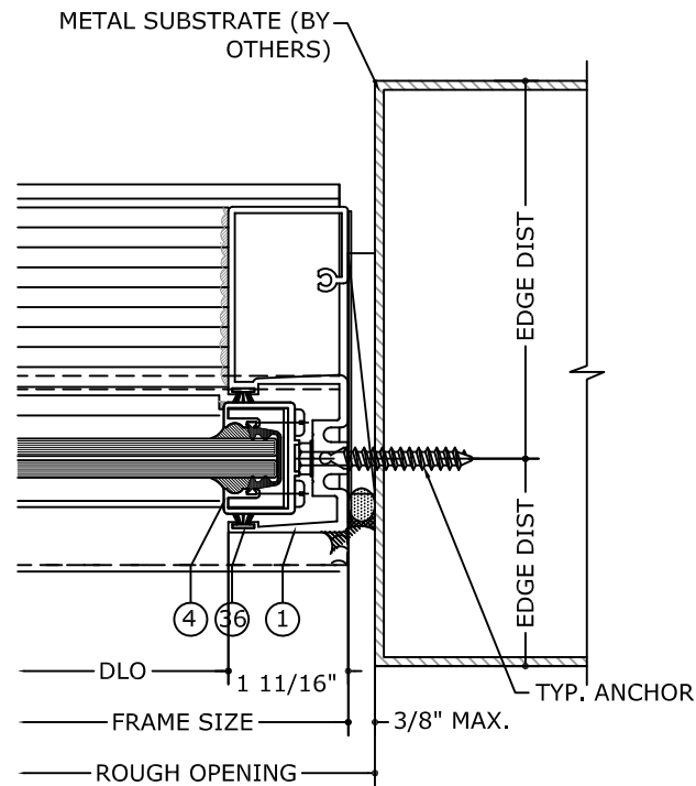
3.6 FIXED JAMB DETAIL (METAL) N.T.S.
