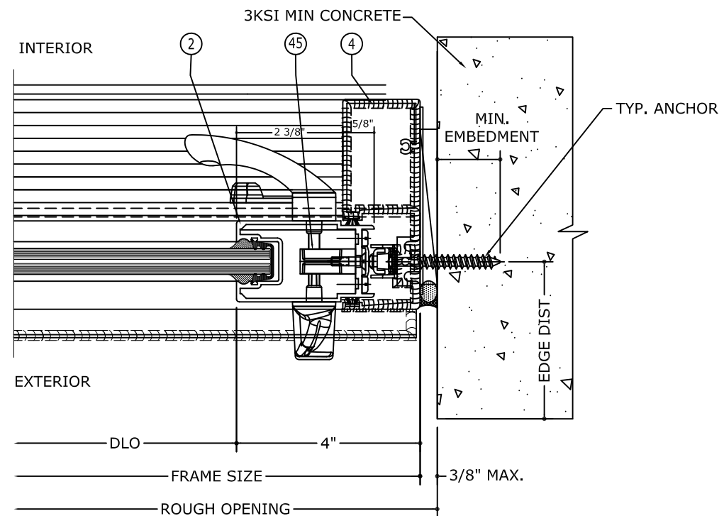
4.1 OPERABLE JAMB DETAIL (CONCRETE) N.T.S
