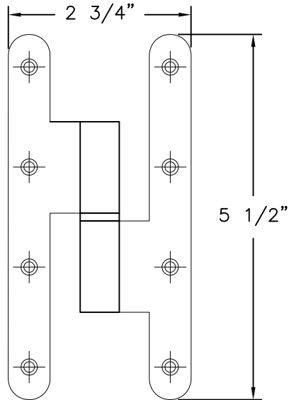
HINGES TYPE FO LASER FROM FAURE ET FILS
