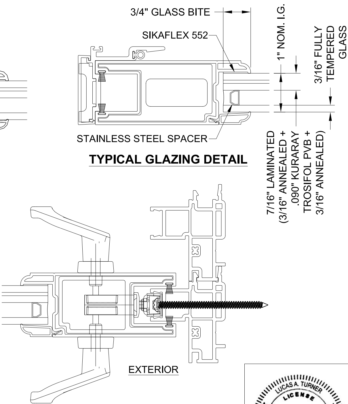
OPERABLE JAMB
