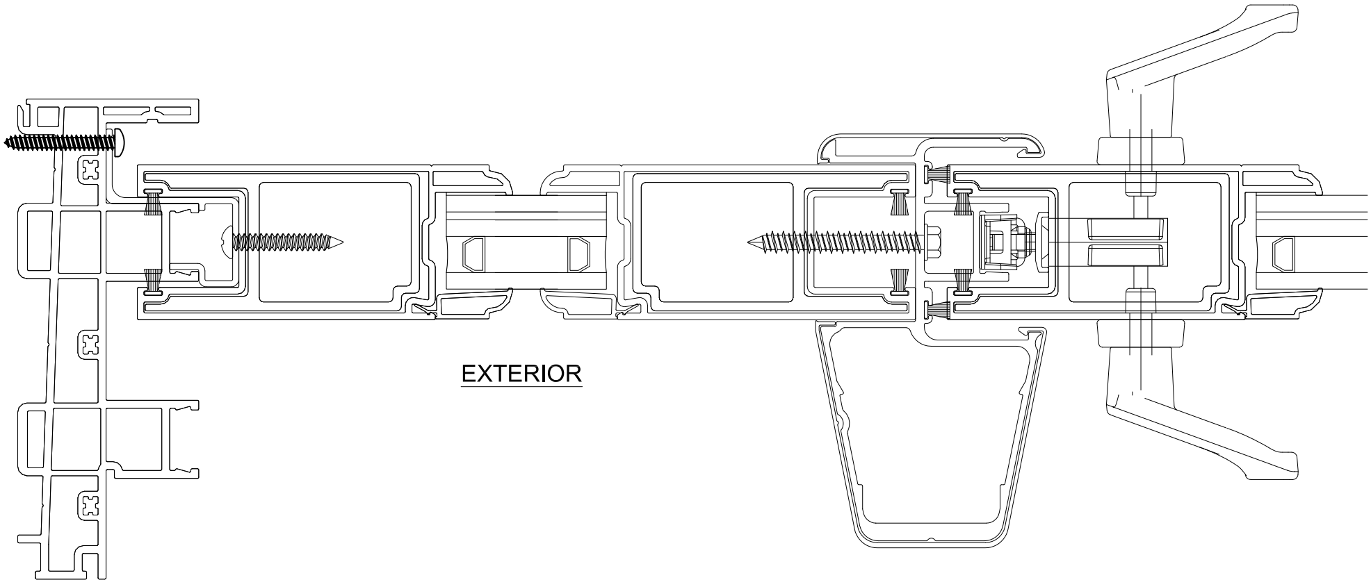
FIXED JAMB
