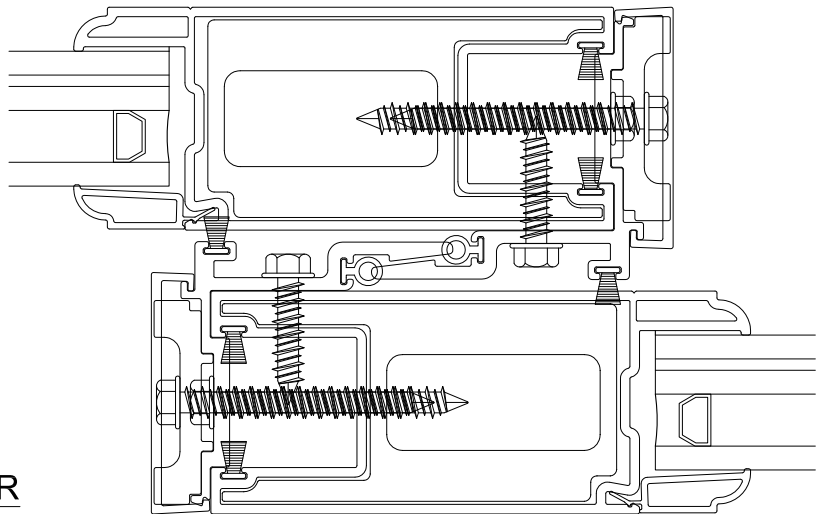
INTERLOCK
