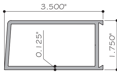
10 DOOR JAMB STILE WW1315 (6063-T5)
