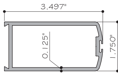
11 DOOR ASTRAGAL WW1316 (6063-T5)
