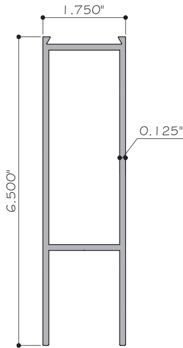
9 DOOR BOTT. RAIL WW1314 (6063-T5)
