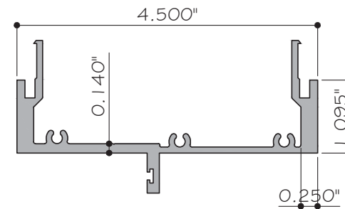
4 JAMB FOR DOOR WW17J (6063-T5)
