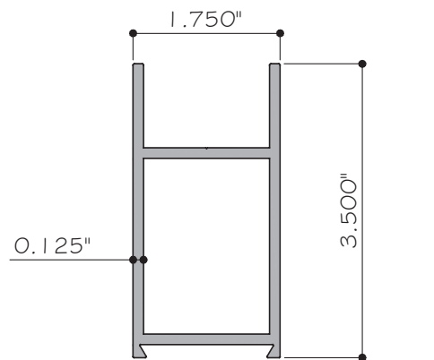
8 DOOR TOP RAIL WW1311 (6063-T5)
