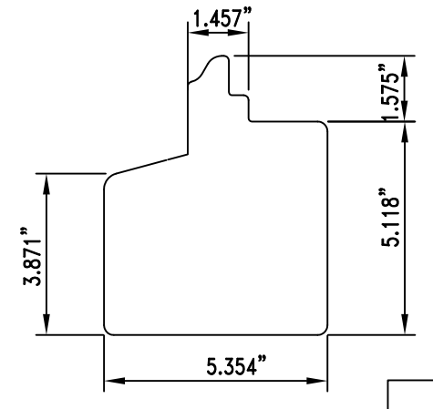
2 SILL Scale: 1/2 FULL SIZE
