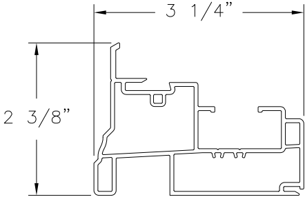
JAMB EXTRUDED PVC (10002932)
