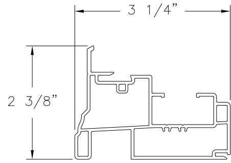
JAMB EXTRUDED PVC (10002932)
