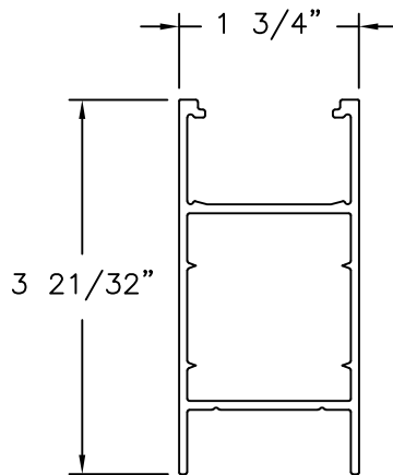
DOOR RAIL ALUMINUM 6063-T5
