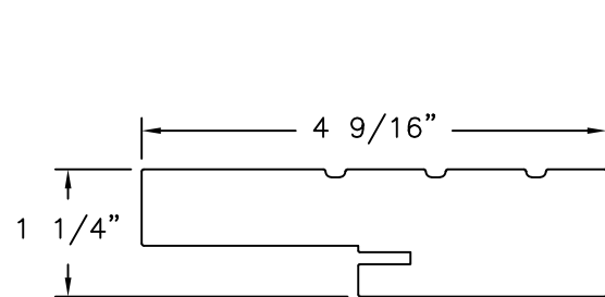
HEAD FRAME & JAMB COMPOSITE
