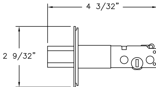
DOOR DEADBOLT STEEL (KWIKSET 980)
