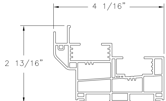
JAMB FRAME VINYL PVC (10005083)
