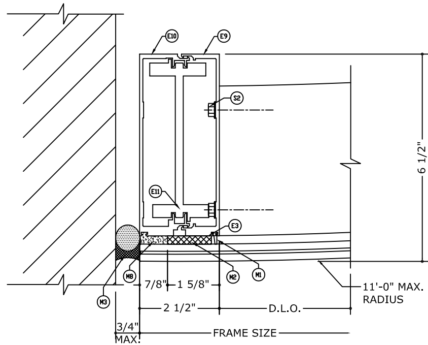
13 JAMB DETAIL N.T.S
