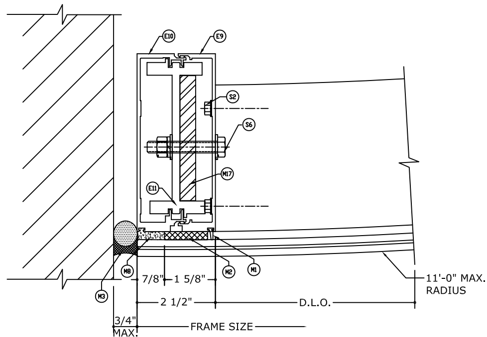
15 JAMB DETAIL N.T.S
