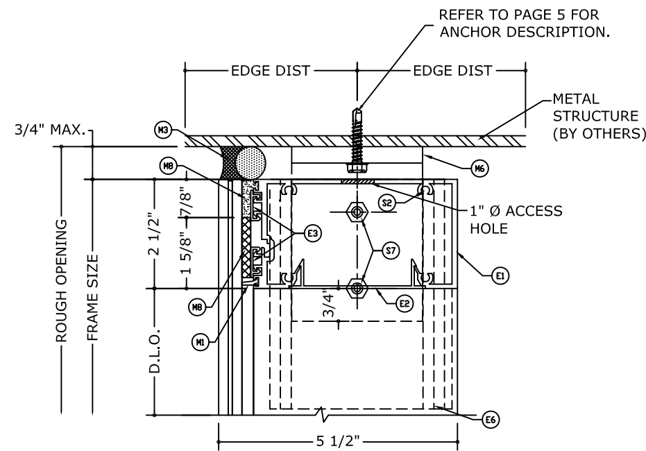
1.1 HEAD DETAIL (METAL) N.T.S
