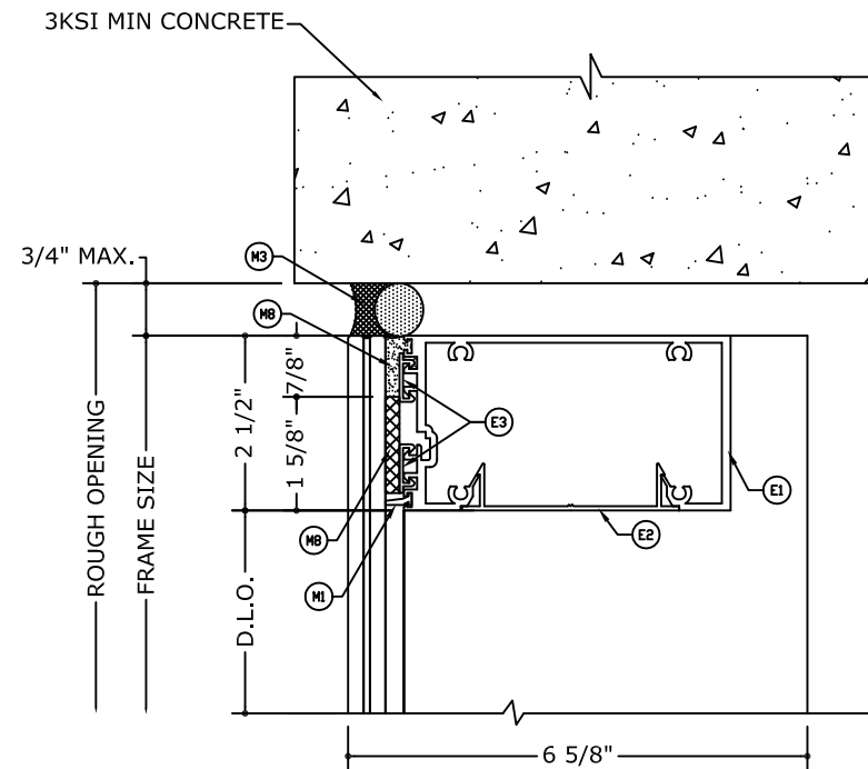
1.2 HEAD DETAIL N.T.S
