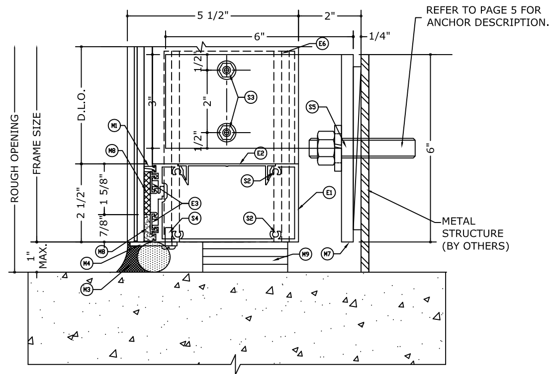
2.1 SILL DETAIL (METAL) N.T.S
