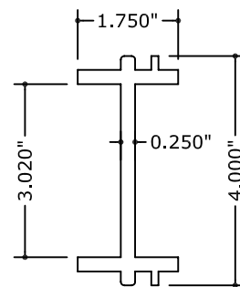
E6 ALUMINUM SPLICER
