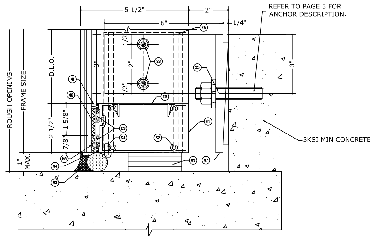
2 SILL DETAIL (CONCRETE) N.T.S
