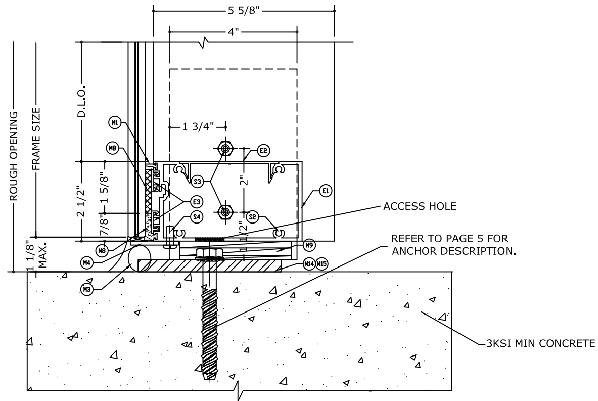
2.2 SILL DETAIL (CONCRETE) N.T.S
