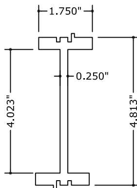
E11 ALUMINUM SPLICER
