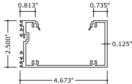
E1 HEAD / SILL / HORIZONTAL
