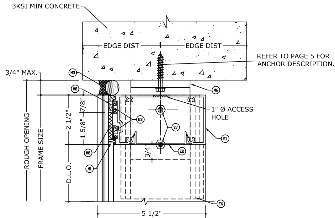
1 HEAD DETAIL (CONCRETE) N.T.S
