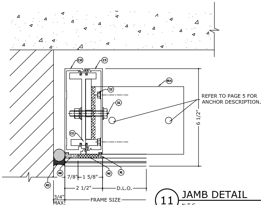
9 JAMB DETAIL N.T.S
