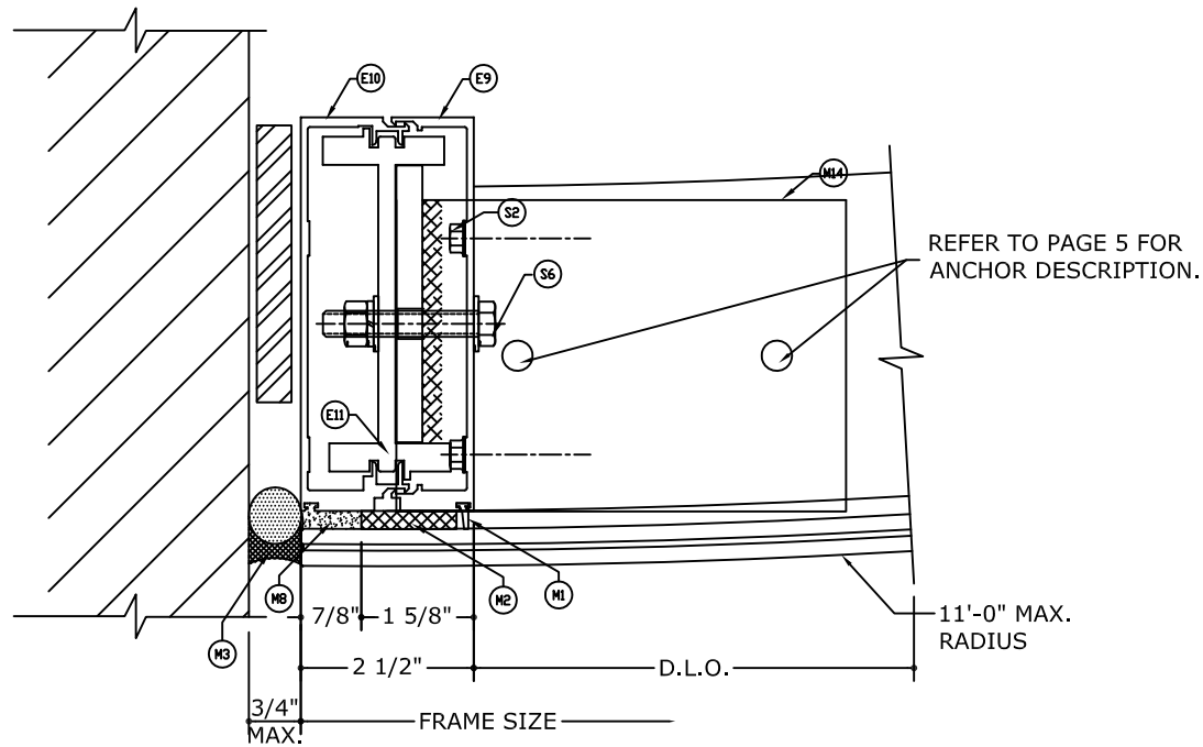
17 JAMB DETAIL N.T.S
