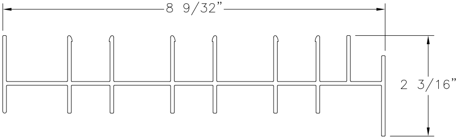
FRAME JAMB 3TRACK, FLANGE ALUMINUM 6005-T5 (M-2529)
