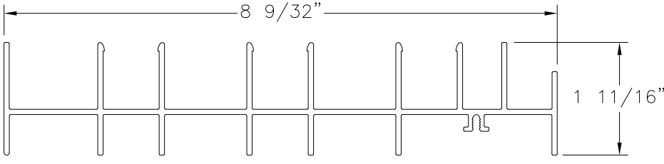
FRAME JAMB 3TRACK, FINLESS ALUMINUM 6005-T5 (M-2523)
