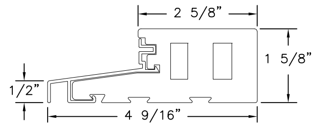
DOOR SILL
