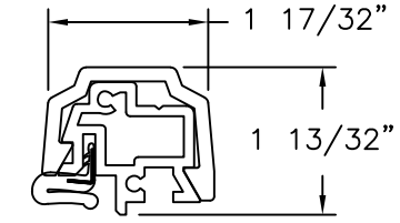
T-ASTRAGAL RIGID PVC
