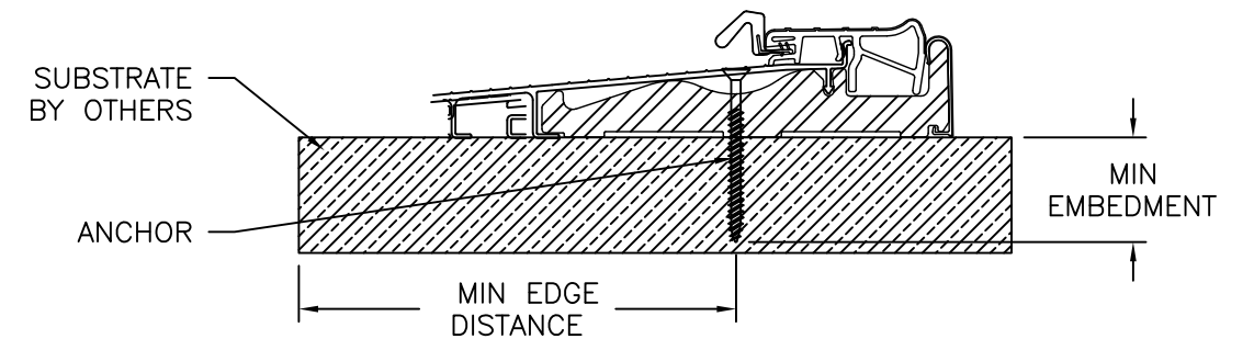
ENDURA ADA THRESHOLD ZOBLH7815
