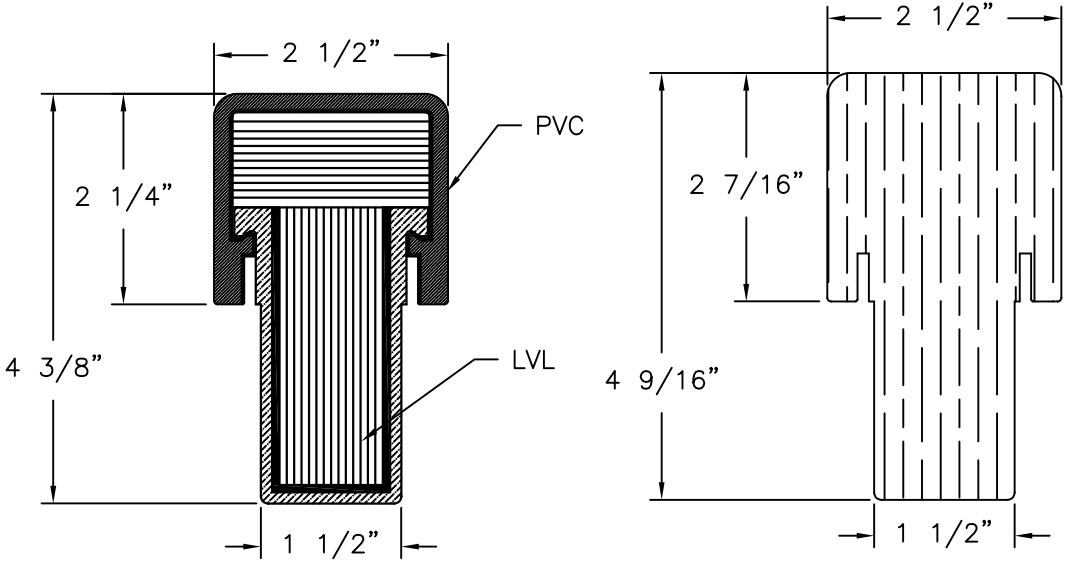
T-MULLION
