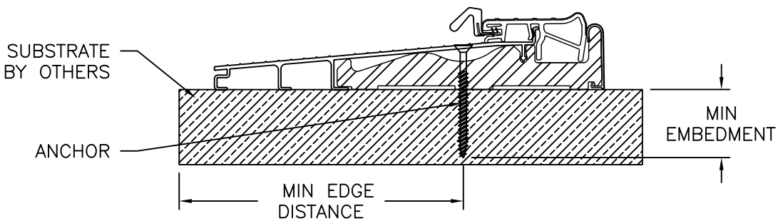
ENDURA ADA THRESHOLD ZOBLH7815
