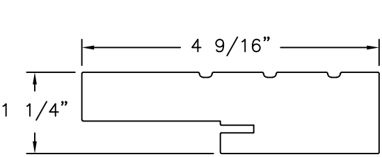
HEAD FRAME & JAMB COMPOSITE
