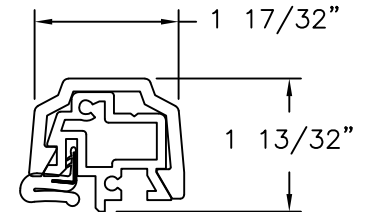
T-ASTRAGAL RIGID PVC
