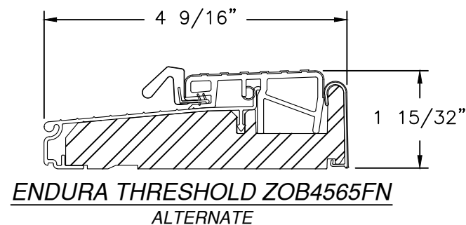
DOOR SILL
