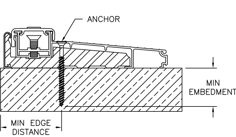
COLUMBIA THRESHOLD ESCON-34
