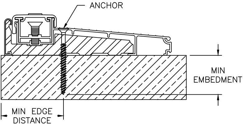
COLUMBIA THRESHOLD ESCON-34
