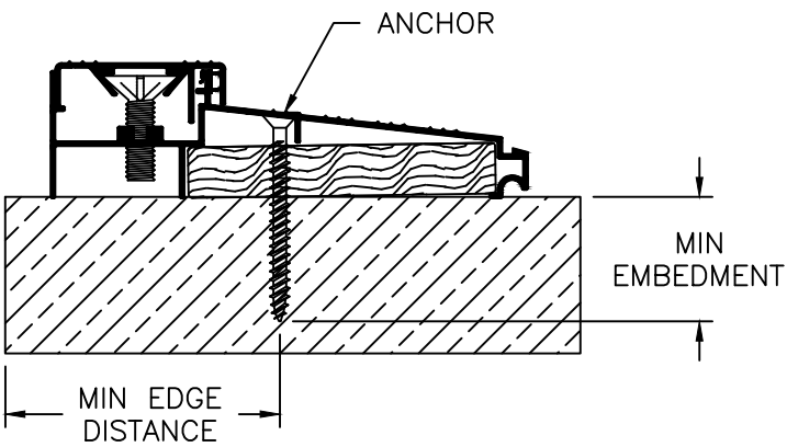
DLP THRESHOLD ISCS
