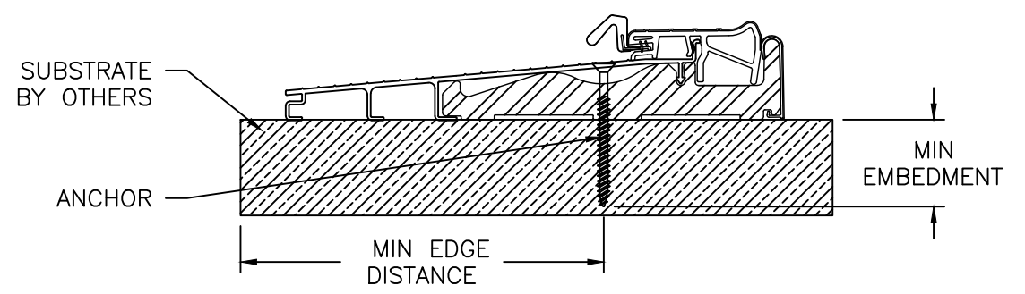
ENDURA ADA THRESHOLD ZOBLH7815
