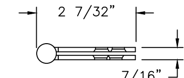
4\" X 4\" DOOR HINGE STEEL
