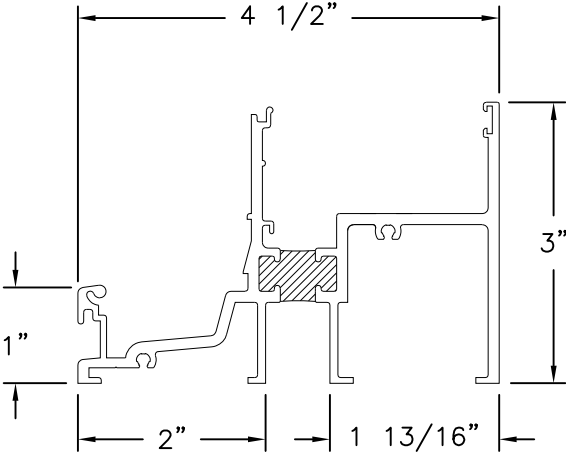
SILL EXTRUSION PW801 ALUMINUM 6063-T5
