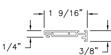
JAMB ISOLATOR STRUT WH809 RIGID PVC
