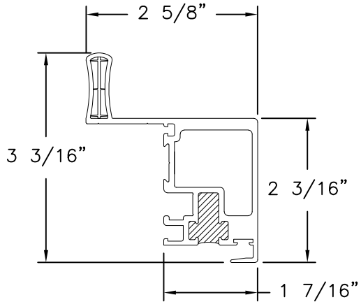
INTERLOCKER HS854 ALUMINUM 6063-T5
