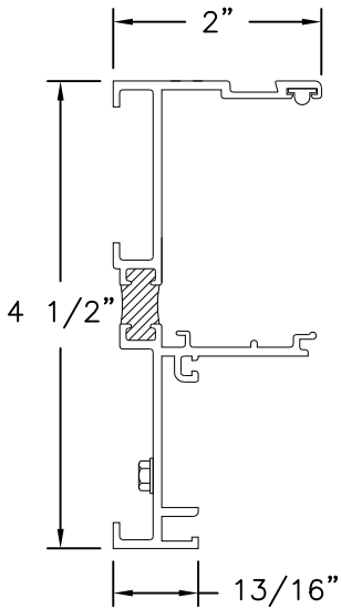
JAMB EXTRUSION HS864 ALUMINUM 6063-T5
