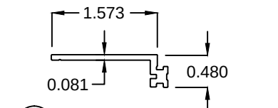
9 FLANGE
