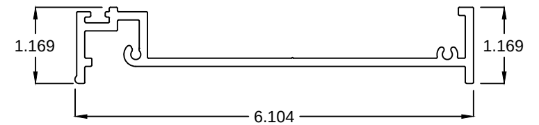
3 SIDE JAMB
