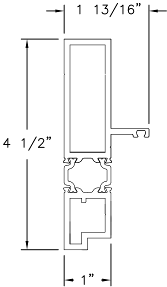
FRAME JAMB JI450 ALUMINUM 6063-T5
