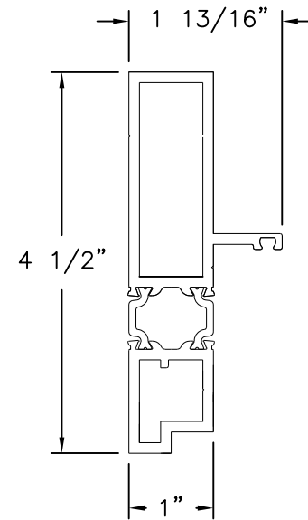
FRAME JAMB JI450 ALUMINUM 6063-T5
