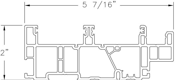
JAMB (7004) RIGID PVC
