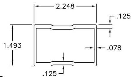
INTERLOCK STIFFENER
