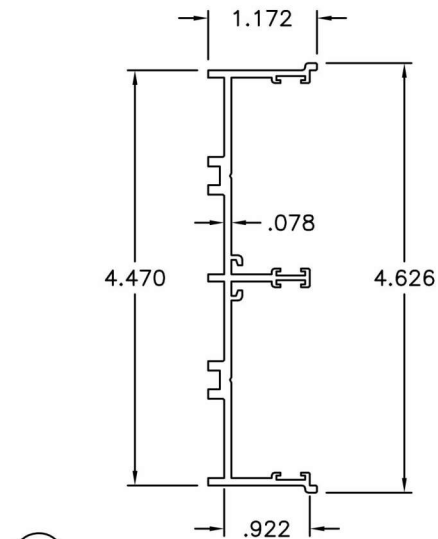
FRAME JAMB
