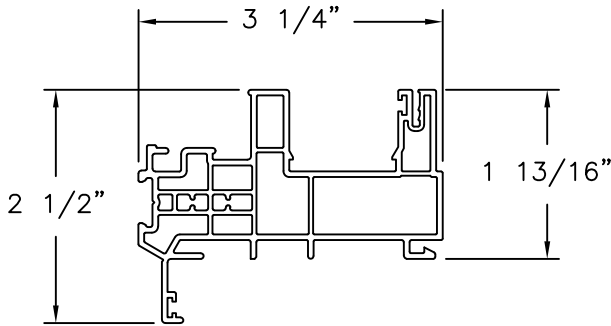
STORM JAMB
