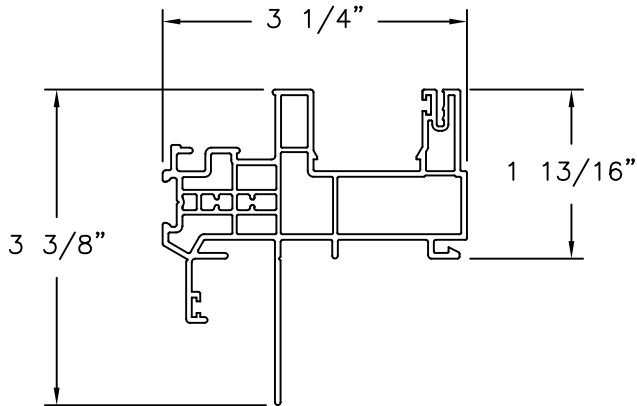
STORM JAMB FIN INSTALLATION
