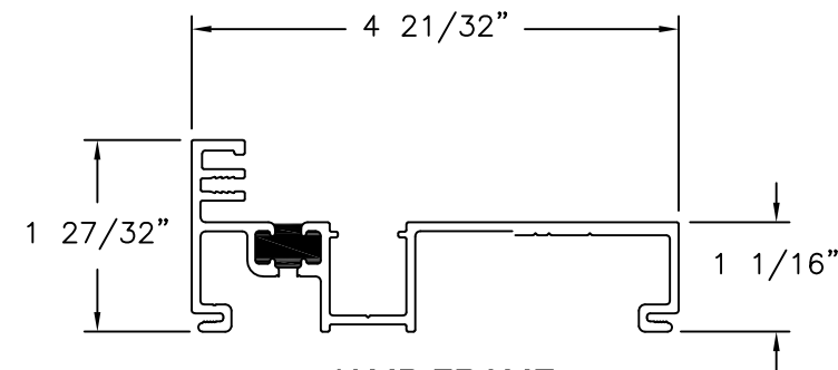
JAMB FRAME ALUMINUM 6063-T5
