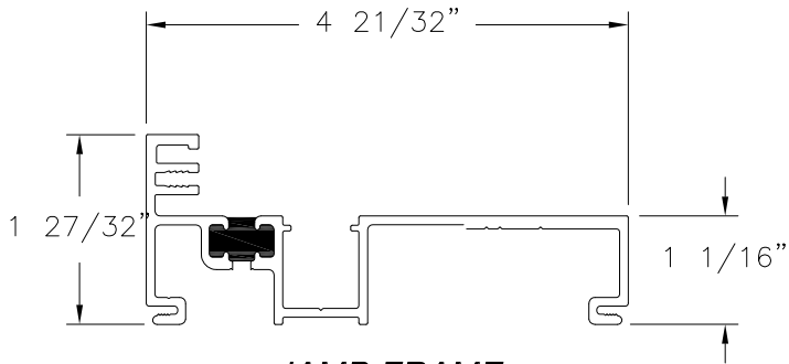
JAMB FRAME ALUMINUM 6063-T5
