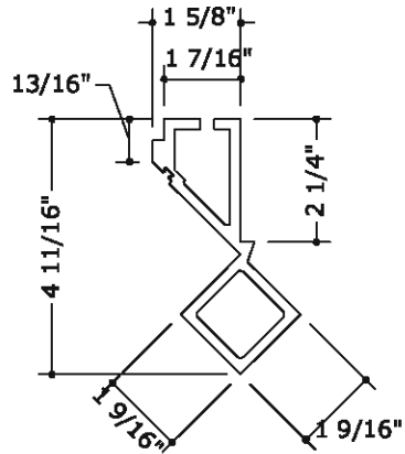
75 90° CORNER CAP
