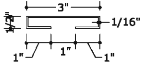
70 EXTERIOR CAP
