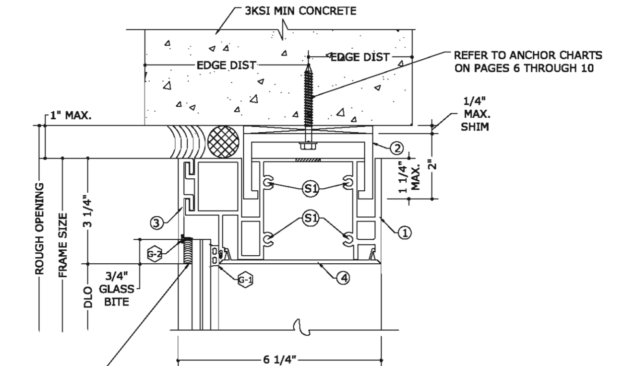
1.1 HEAD DETAIL (CONCRETE) N.T.S
