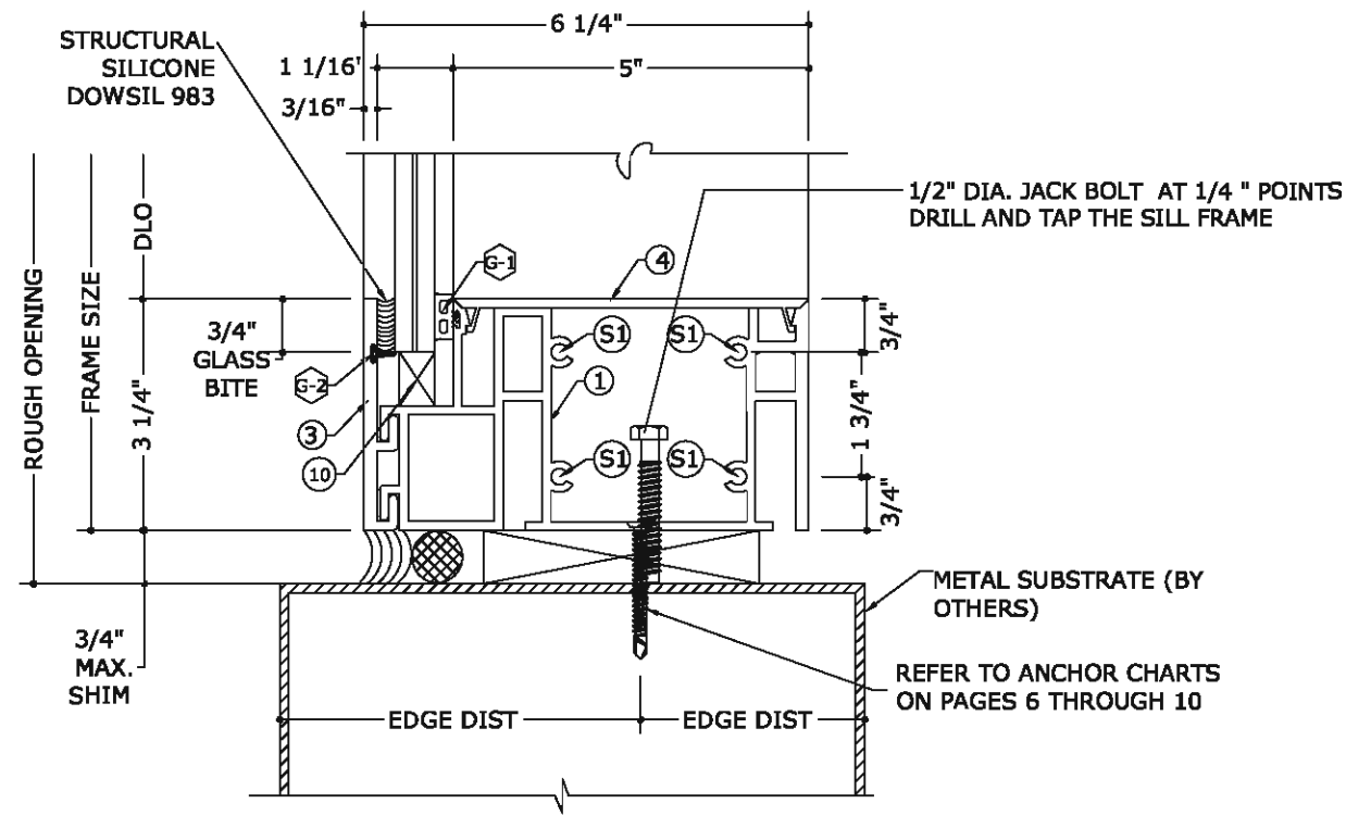
2.3 SILL DETAIL (METAL) N.T.S
