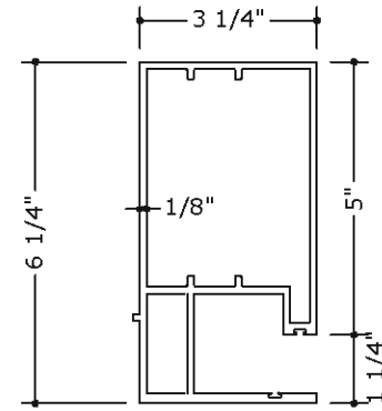
7 JAMB
