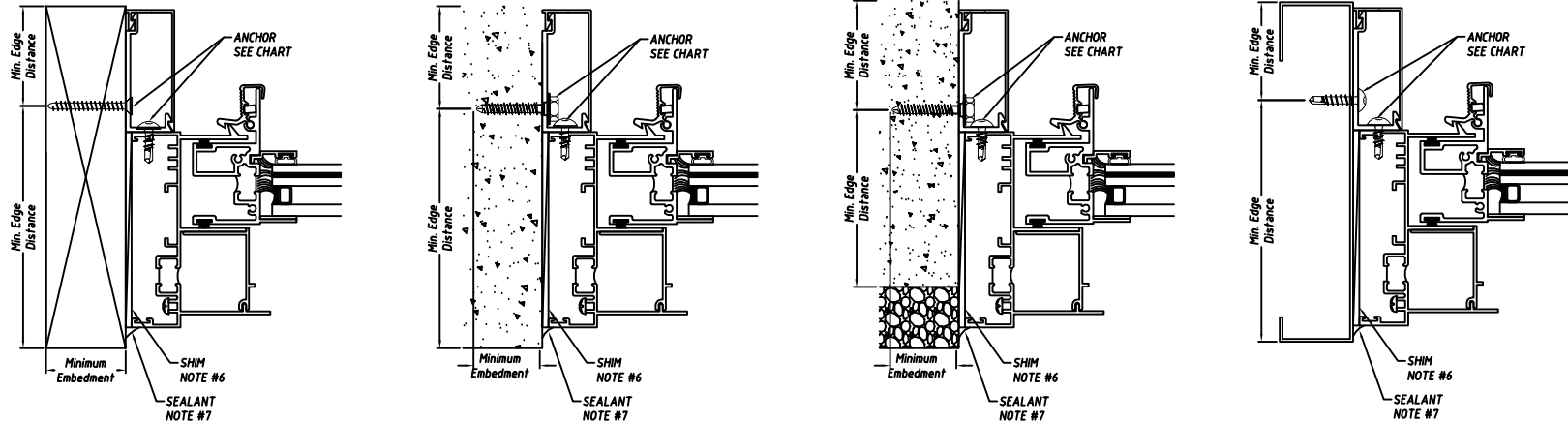
JAMB
