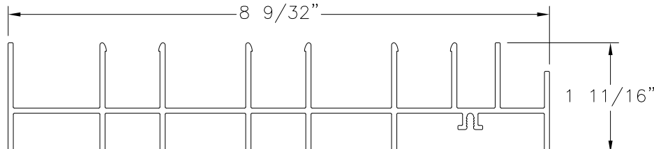
FRAME JAMB 3TRACK, FINLESS ALUMINUM 6005-T5 (M-2523)
