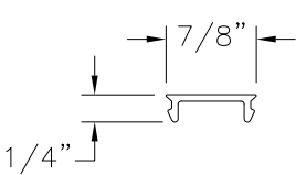
HEAD/JAMB FILLER ALUMINUM 6063-T5 (M-2512)
