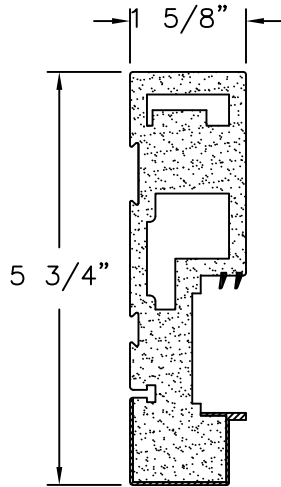
SIDE JAMB FOAM PVC
