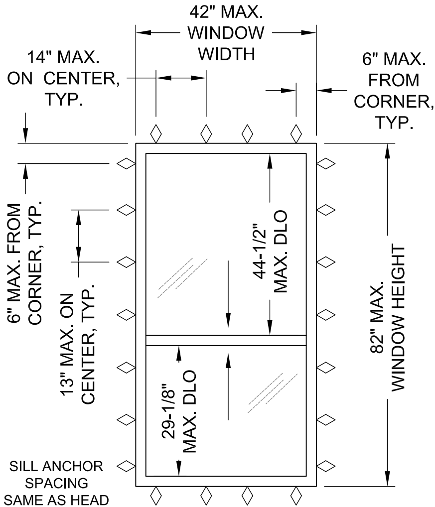
42"x82" ORIEL ELEVATION
