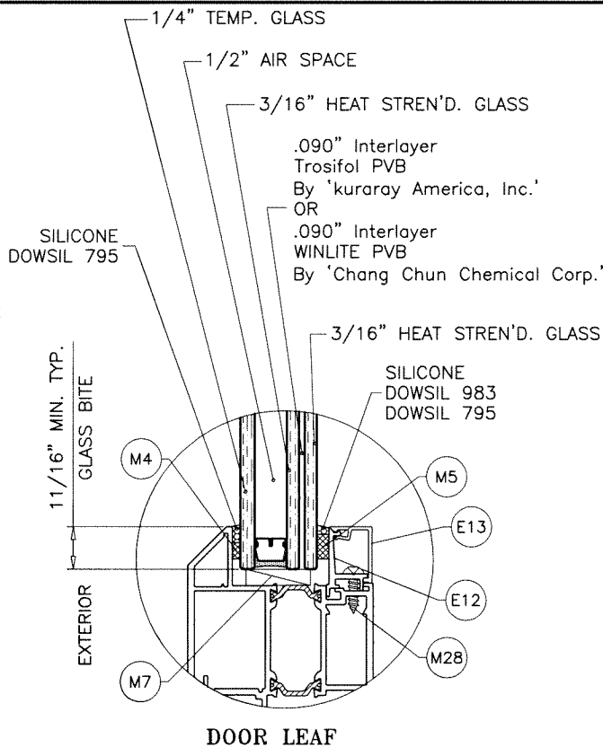
DOOR LEAF
