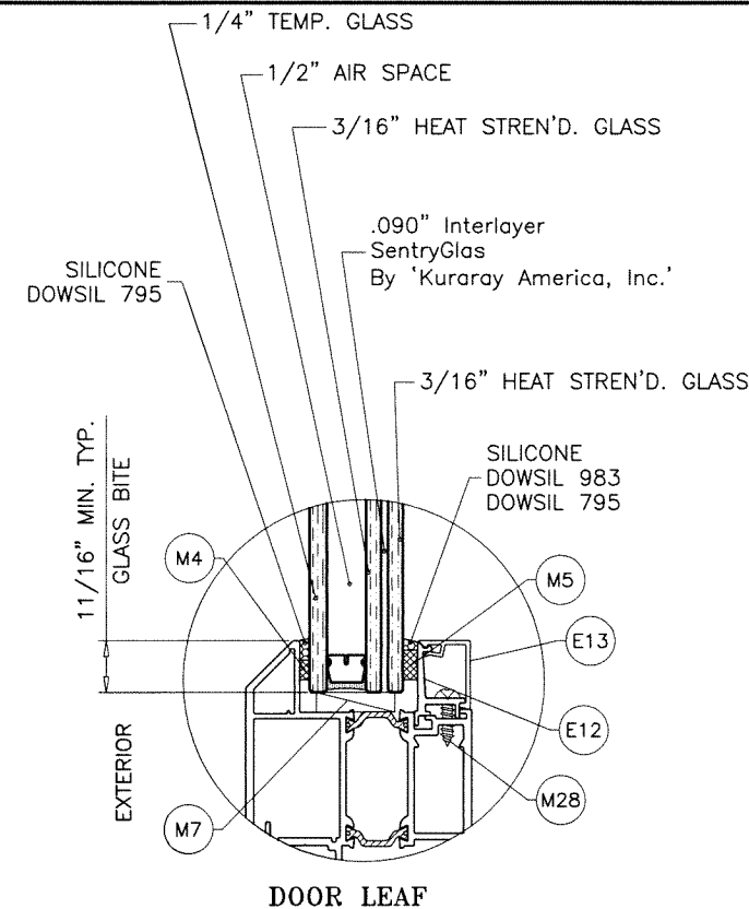
DOOR LEAF
