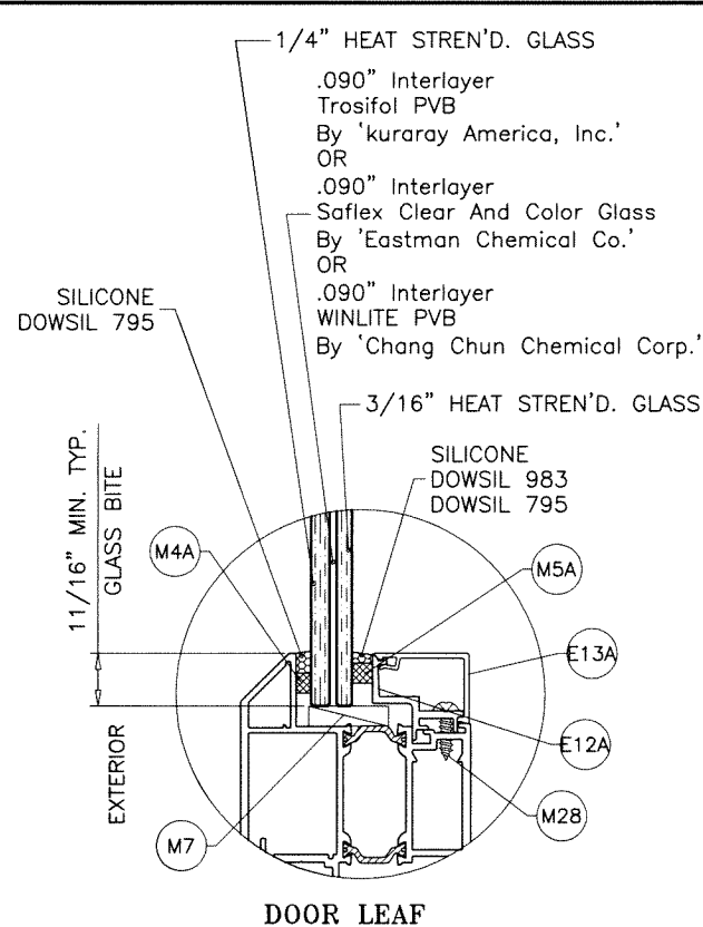
DOOR LEAF
