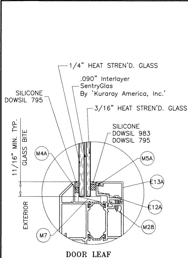
DOOR LEAF
