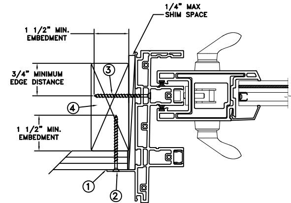
FRAME JAMB SECTION (TYP)
