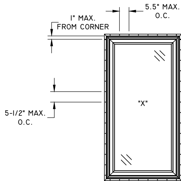
ANCHOR LAYOUT FIN
