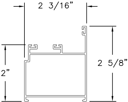
JAMB FRAME ALUMINUM 6063-T6 (MD45003)
