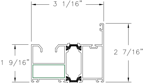
BOTTOM TRACK ALUMINUM 6063-T5 (MD80002)
