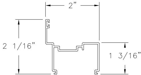
JAMB EXTENDER ALUMINUM 6063-T6 (MD45014)
