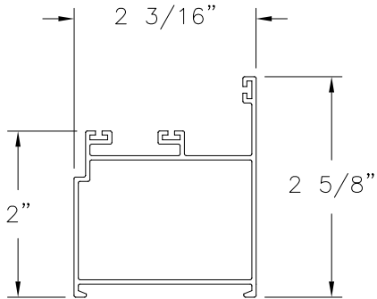
JAMB FRAME ALUMINUM 6063-T6 (MD45003)
